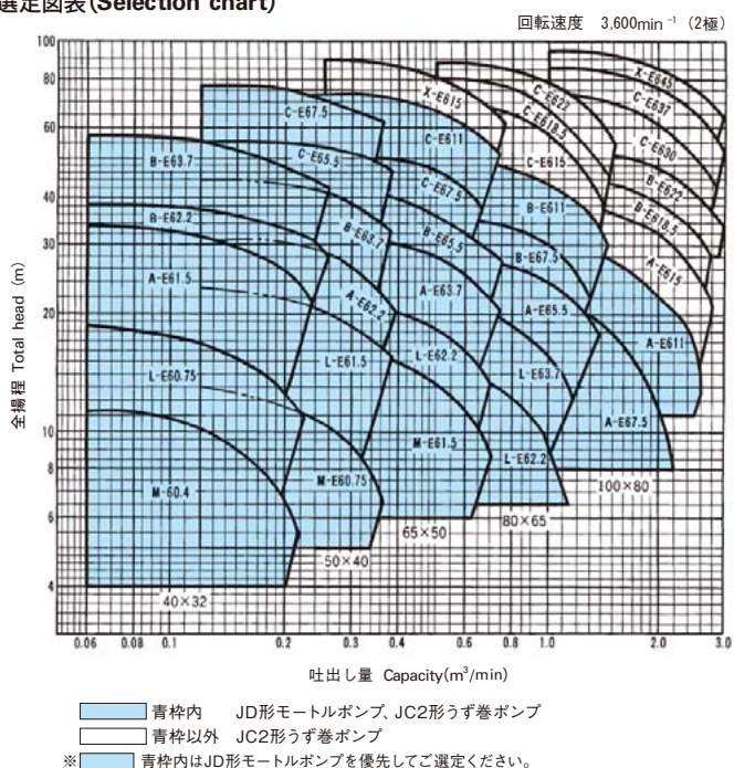
JC2形うず巻ポンプ
