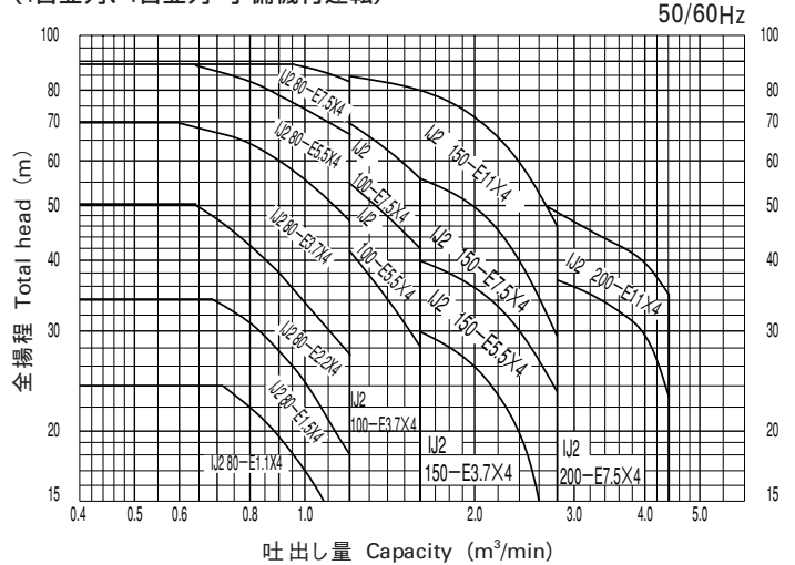
(4台並列、4台並列・予備機付運転)
