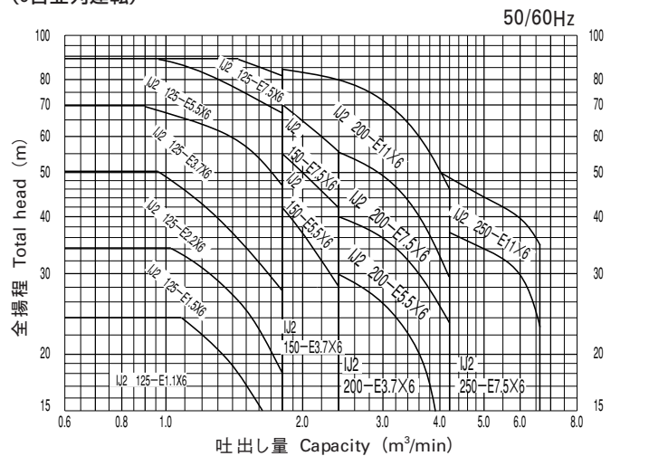
(6台並列運転)
