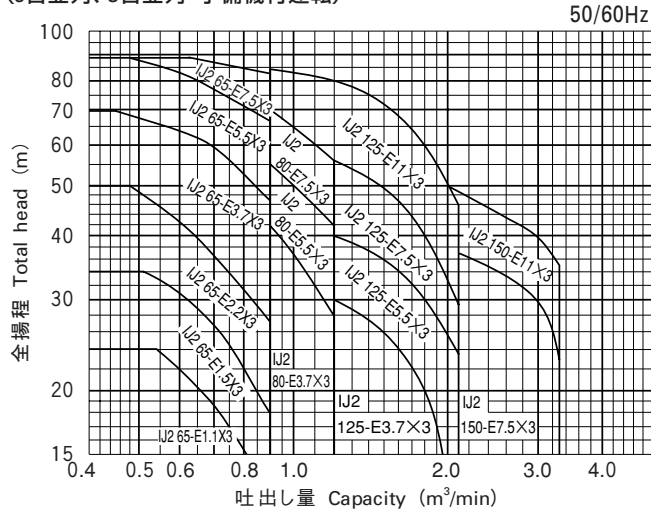
(3台並列、3台並列・予備機付運転)
