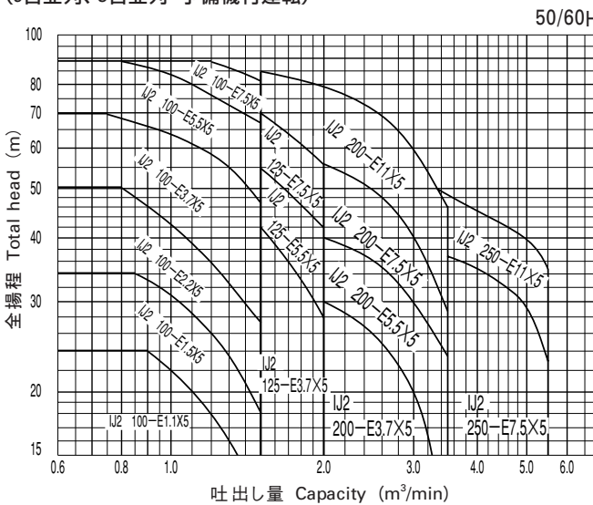
(5台並列、5台並列・予備機付運転)
